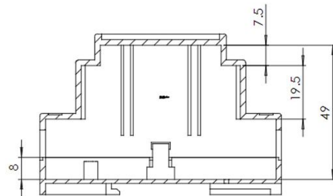
剖面 A-A
