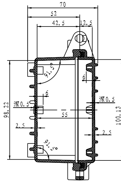
截面 A-A
