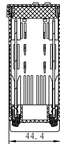
剖面 A-A
