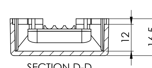
SECTION D-D
