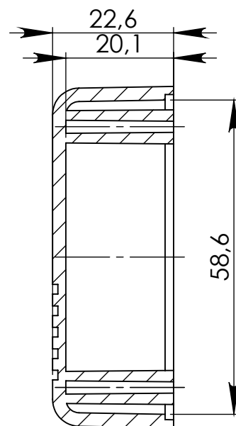
PRZĘKRÓJ B-B
