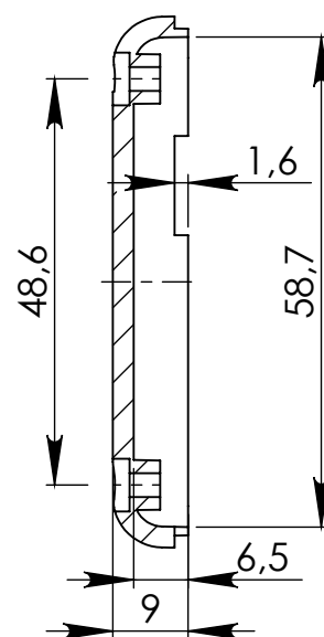
PRZĘKRÓJ A-A
